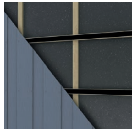
Verticale installatie op houten achterconstructie
