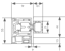
Muurbevestiging 44 mm
