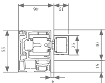
Muurbevestiging 40 mm
