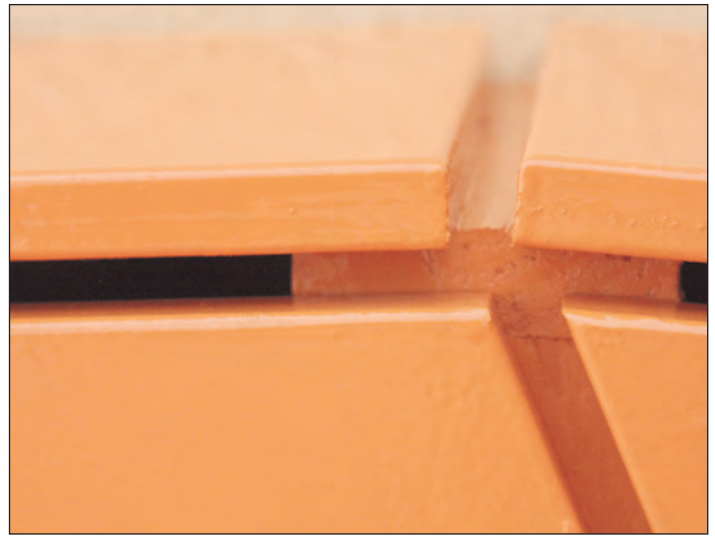
Afbeelding 1. Voorbeeld van goed afronden, ventileren en dilateren van plaatmateriaal.
