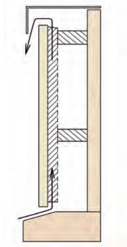
Figuur 3. Schematische voorstelling van de juiste wijze van ventileren.
