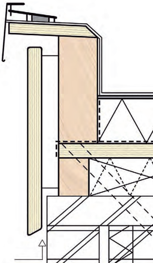
Figuur 8. Voorbeeld aanbrengen van een boeiboord
