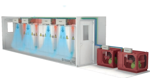
Fig. 2: principio de funcionamiento del climatizador de grúa serie V
