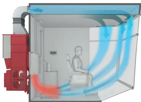
Fig. 1: principio de funcionamiento del climatizador de grúa serie T
