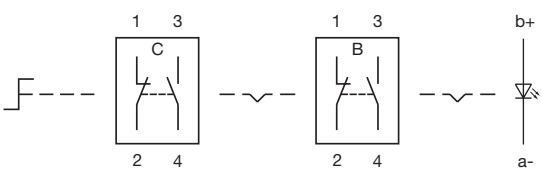
Wiring diagram 285
