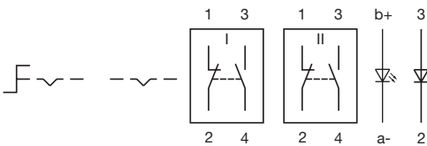
Wiring diagram 283
