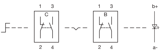
Wiring diagram 285
