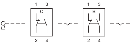
Wiring diagram 259
