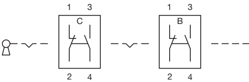
Wiring diagram 261
